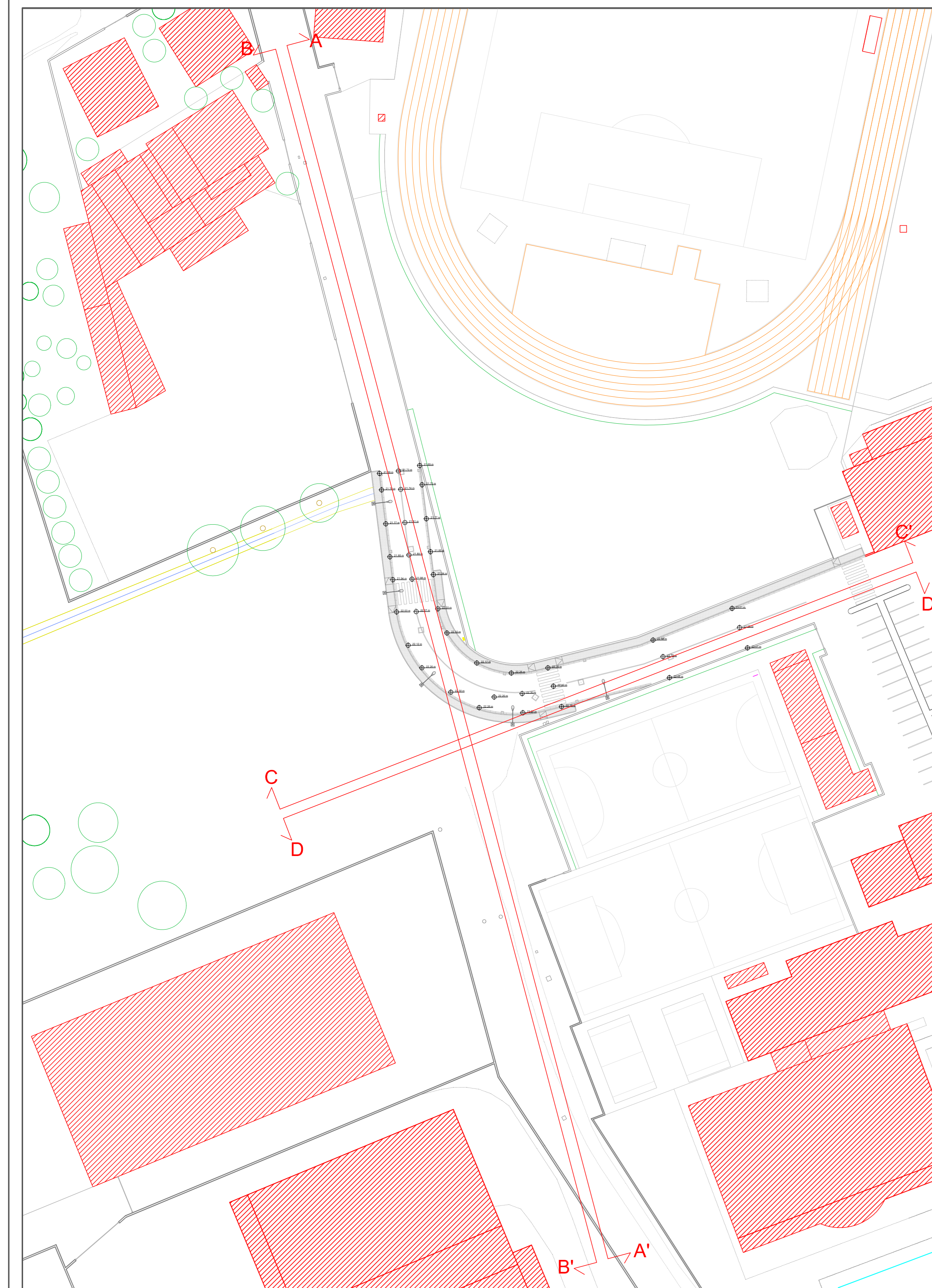
INQUADRAMENTO 1:500
